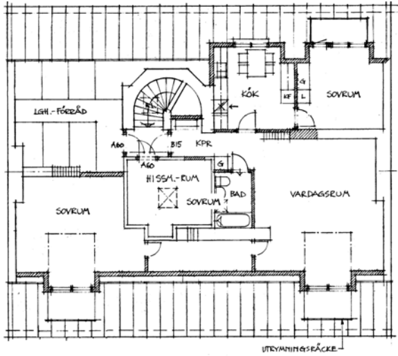
Vindsvåning
