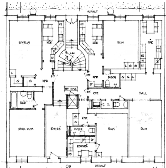
Bottenvåning
