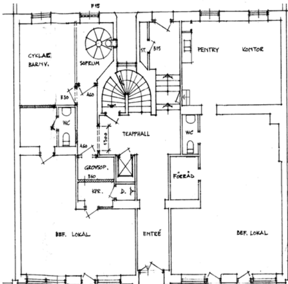
Gatuplan
