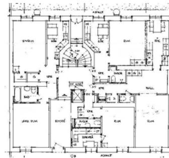
Bottenvåning
