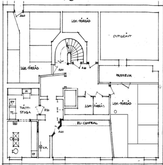
Källarplan
